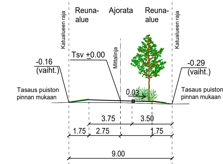
TYYPPIPOIKKILEIKKAUS GRETASBÄCKINTIE PL180 1:200
