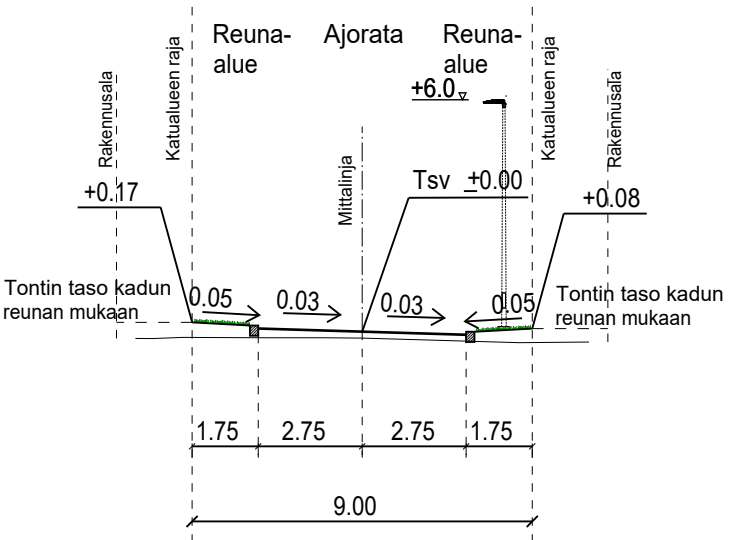
TYYPPIPOIKKILEIKKAUS GRETASBÄCKINTIE PL30 1:200
