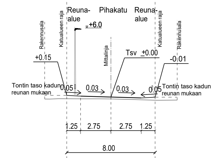
TYYPPIPOIKKILEIKKAUS GRETASBÄCKINTIE PL-4.0 1:200
