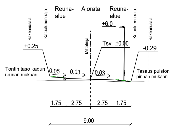
TYYPPIPOIKKILEIKKAUS GRETASBÄCKINTIE PL100 1:200
