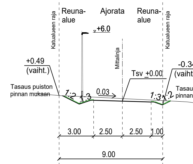
TYYPPIPOIKKILEIKKAUS POHJANMETSÄNREUNA PL 340 1:200
