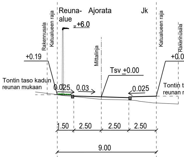
TYYPPIPOIKKILEIKKAUS POHJANMETSÄNREUNA PL 240 1:200
