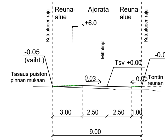
TYYPPIPOIKKILEIKKAUS POHJANMETSÄNREUNA PL 310 1:200
