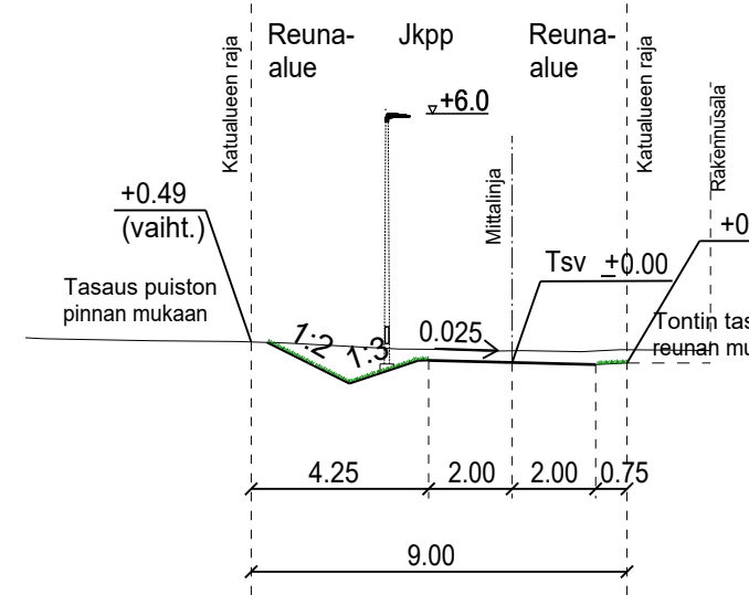
TYYPPIPOIKKILEIKKAUS POHJANMETSÄNREUNA PL 80 1:200
