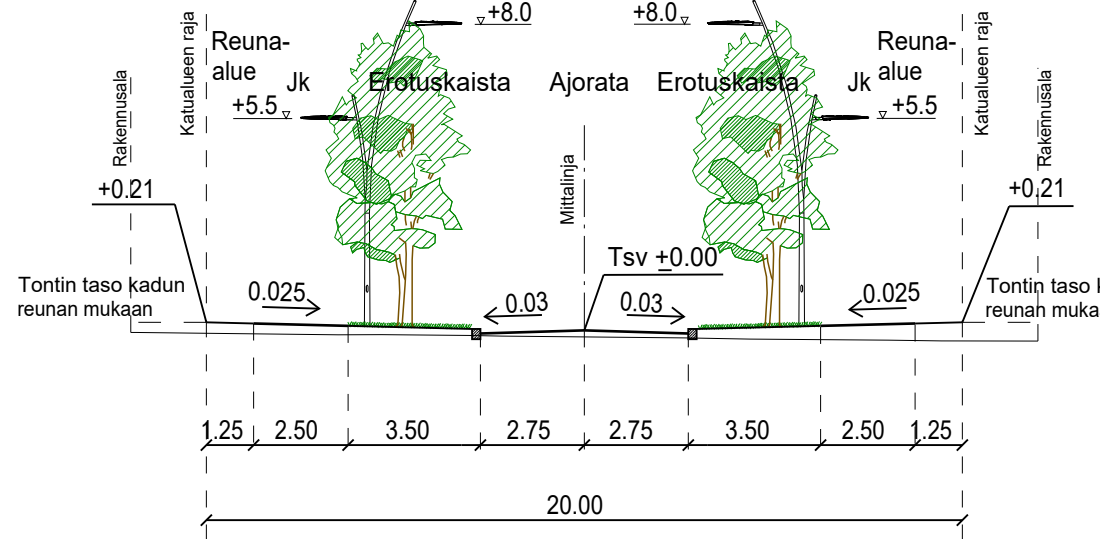
TYYPPIPOIKKILEIKKAUS NIKKILÄN KARTANONTIE PL 130 1:200
