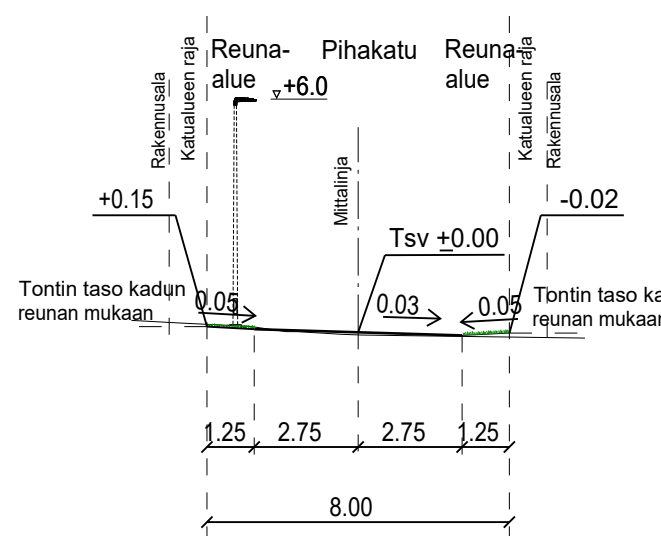
TYYPPIPOIKKILEIKKAUS NIKKILÄN KARTANONTIE PL 30 1:200
