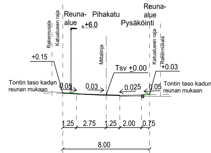
TYYPPIPOIKKILEIKKAUS NIKKILÄN KARTANONTIE PL 130 1:200
