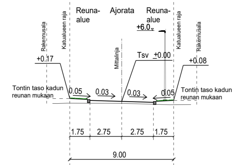
TYYPPIPOIKKILEIKKAUS GRETASBÄCKINTIE PL30 1:200
