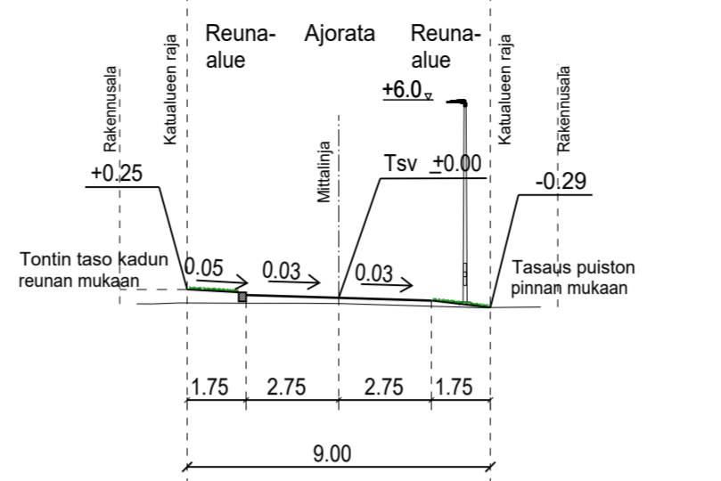
TYYPPIPOIKKILEIKKAUS GRETASBÄCKINTIE PL100 1:200
