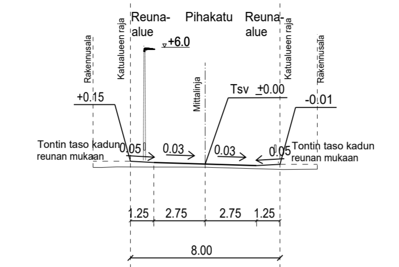
TYYPPIPOIKKILEIKKAUS GRETASBÄCKINTIE PL-4.0 1:200
