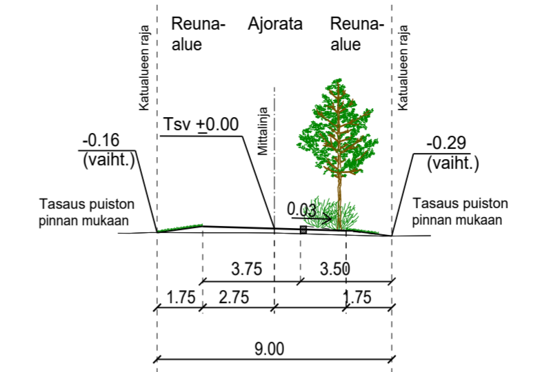
TYYPPIPOIKKILEIKKAUS GRETASBÄCKINTIE PL180 1:200
