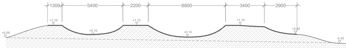
Pituusleikkaus B-B, 1:200
