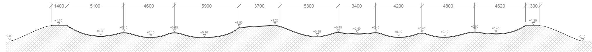
Pituusleikkaus A-A, 1:200
