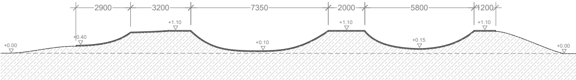
Pituusleikkaus B-B, 1:200
