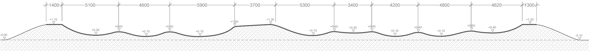
Pituusleikkaus A-A, 1:200
