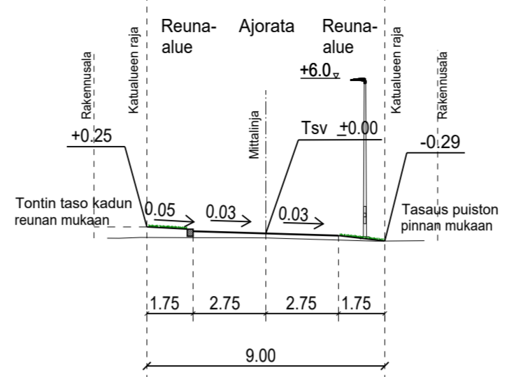
TYYPPIPOIKKILEIKKAUS GRETASBÄCKINTIE PL100 1:200
