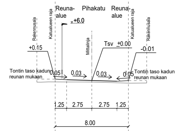
TYYPPIPOIKKILEIKKAUS GRETASBÄCKINTIE PL-4.0 1:200
