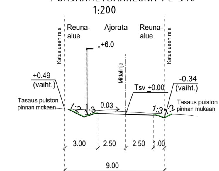
TYYPPIPOIKKILEIKKAUS POHJANMETSÄNREUNA PL 340 1:200
