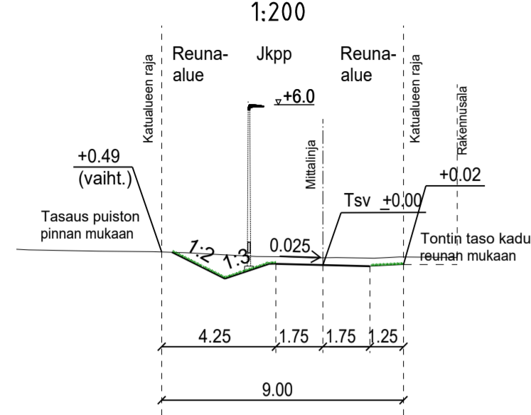
TYYPPIPOIKKILEIKKAUS POHJANMETSÄNREUNA PL 80 1:200
