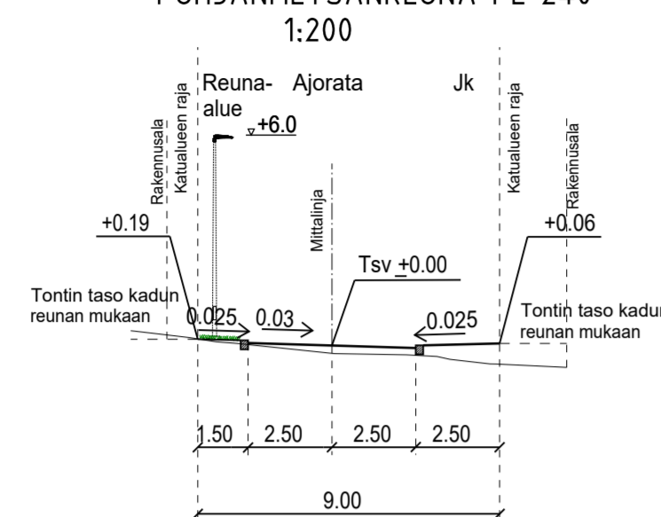
TYYPPIPOIKKILEIKKAUS POHJANMETSÄNREUNA PL 240 1:200
