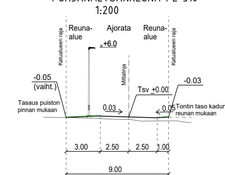
TYYPPIPOIKKILEIKKAUS POHJANMETSÄNREUNA PL 310 1:200
