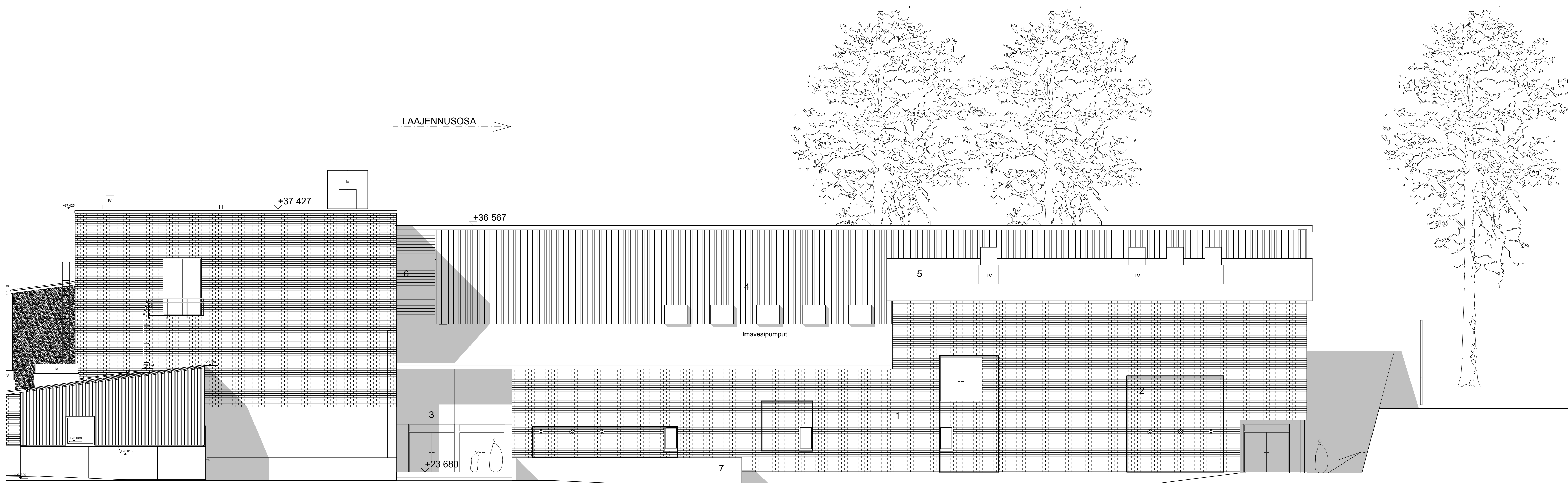
JULKISIVU ITÄÄN 1:100
